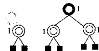
图 3-6 黑高度为 1 的最多红结点红黑树
