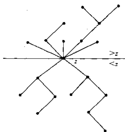
图 2-5 序关系树
