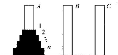
图 2-19 双色 Hanoi 塔
