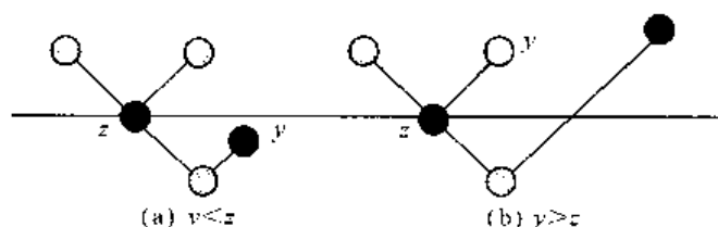
图 2-6 对手策略
