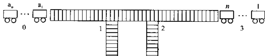
图 5-28 铁路转轨栈
