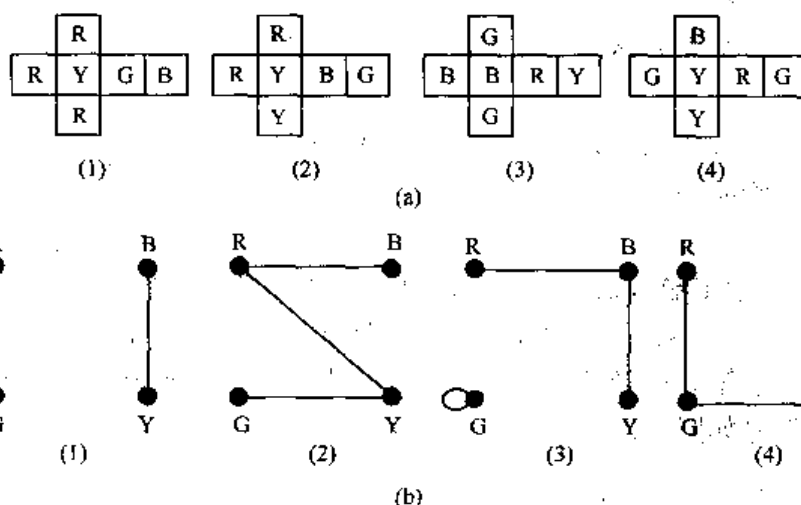
图 5-3 立方体及其相应的子图
